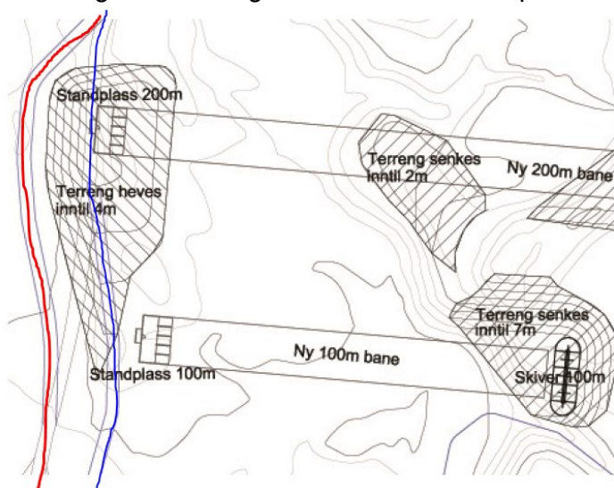
Figur 2: Omlagt atkomst til skytebanen
